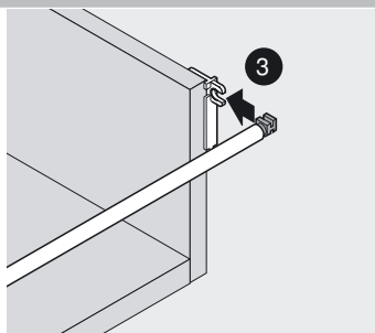
Montage hinten
