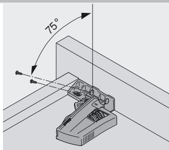
Dreiseitiger Schubkasten
