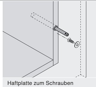
Haftplatte zum Schrauben
