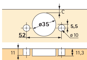
Bohrmaße T43 / Flash
