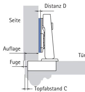
Bohrmaße T42
