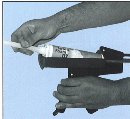
4. In Handdruckpistole einlegen. Ruckhaftes Auspressen vermeiden, sonst Gefahr der Inhomogenität
