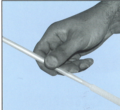
3. Bei Bedarf (enge Fuge bzw. tiefes Futter) Verlängerungsröhrchen auf Mischdüse aufstecken.
