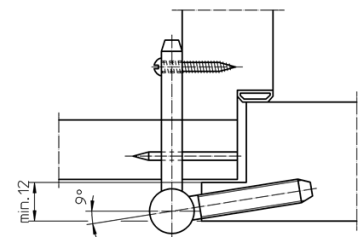
Querschnitt 1
