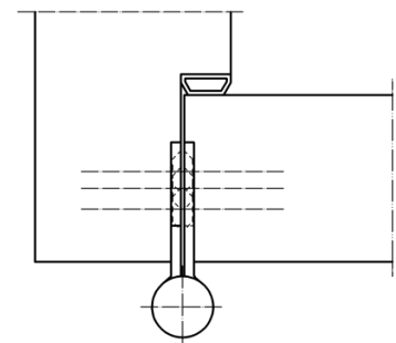
Querschnitt 1
