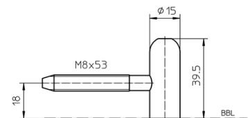
Vorderansicht
