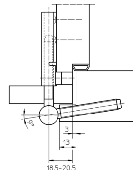
Querschnitt 1
