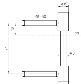
Vorderansicht
