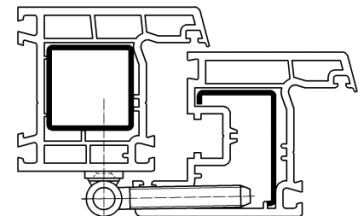
Querschnitt
