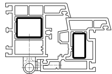
Querschnitt
