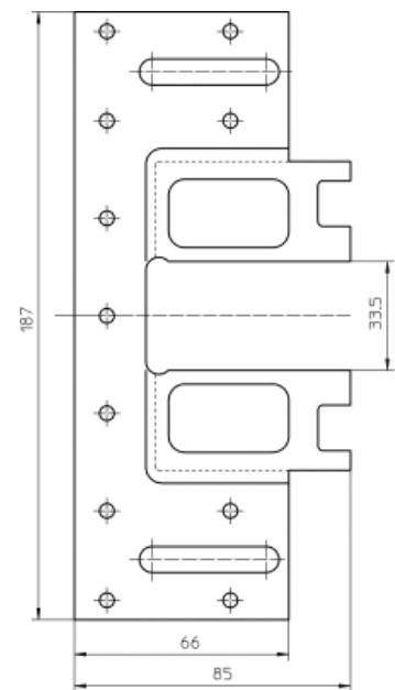
Vorderansicht
